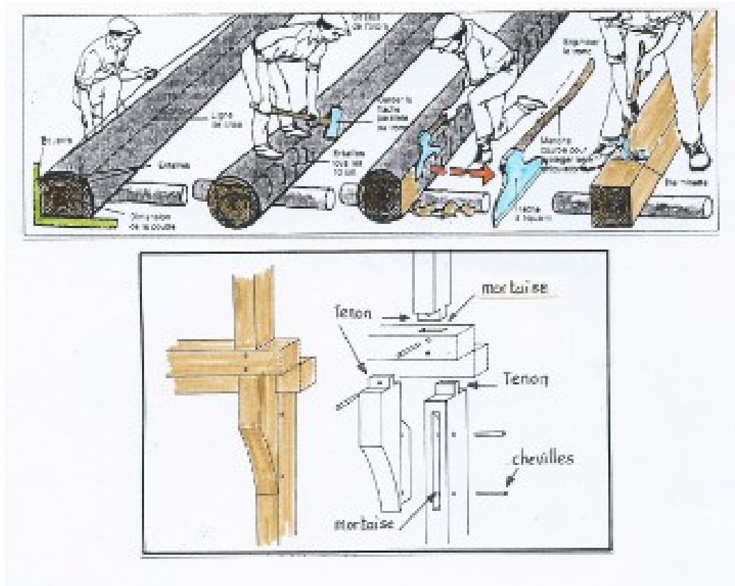
1 - de la grume à l'équarrissage de l'arbre en atelier 2 - Schémas d'assemblages
